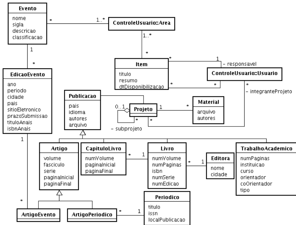
Figura 4.5: Diagrama de classes do pacote ControleItens do Portal do LabES.
