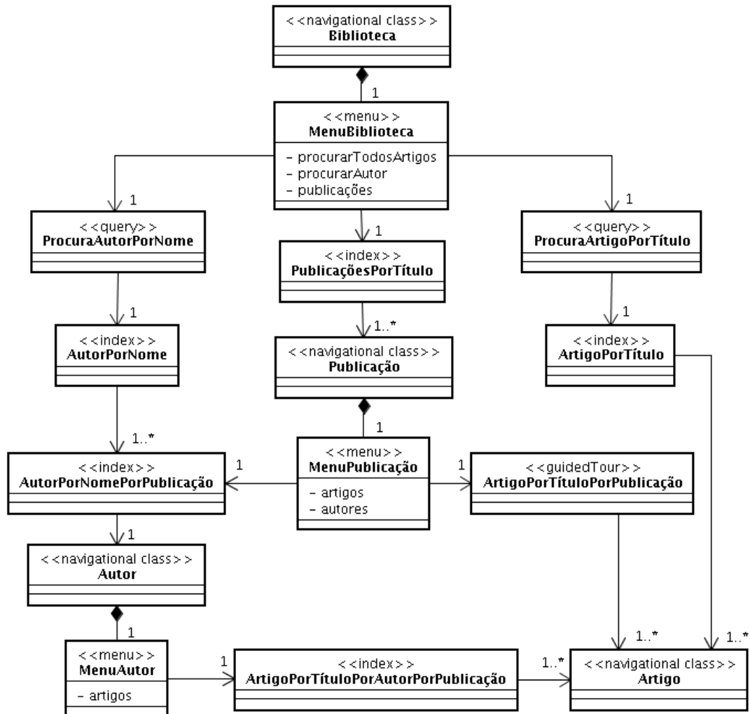
Figura 2.10: Exemplo de modelo de estrutura de navegação em UWE (KOCH et al, 2000)
